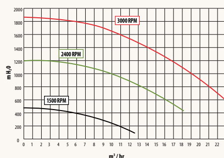
CURVAS DE RENDIMENTO / BOMBA RS II® VSTD 1,5 cv
