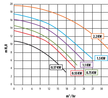
CURVAS DE RENDIMENTO / BOMBA SUPERFLO 50HZ
