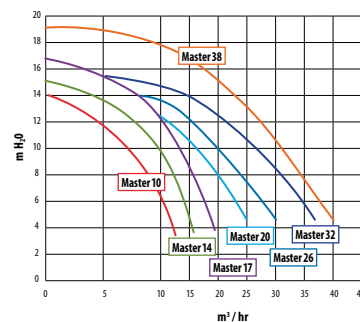
CURVAS DE RENDIMENTO / BOMBA AQUA MASTER
