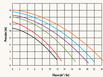
CURVAS DE RENDIMENTO / BOMBA POWERLINE PL
